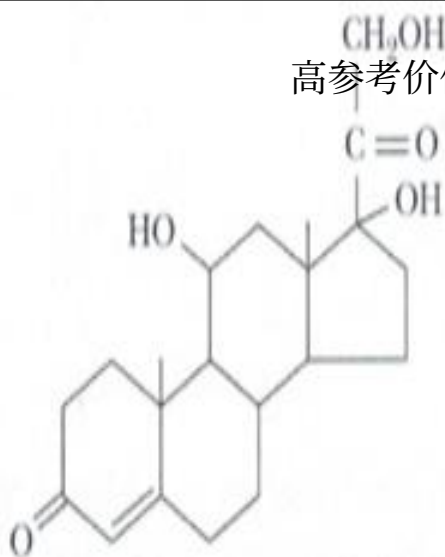
Cortisol
