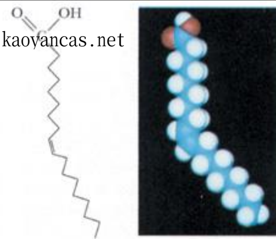
Oleic acid
