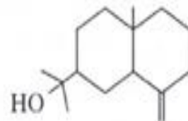
欧倍醇
