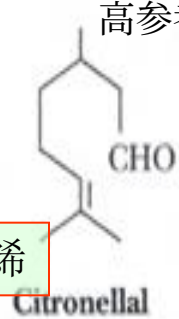
香茅醛
