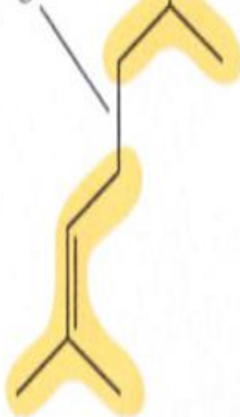
Geraniol
