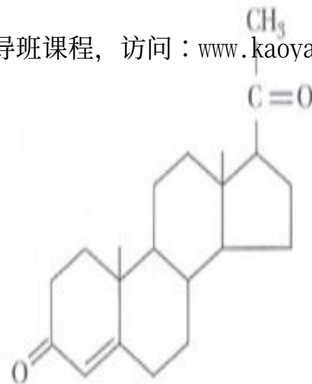
Progesterone
