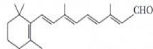
视黄醛
