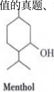
薄荷醇
