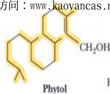
叶绿醇
